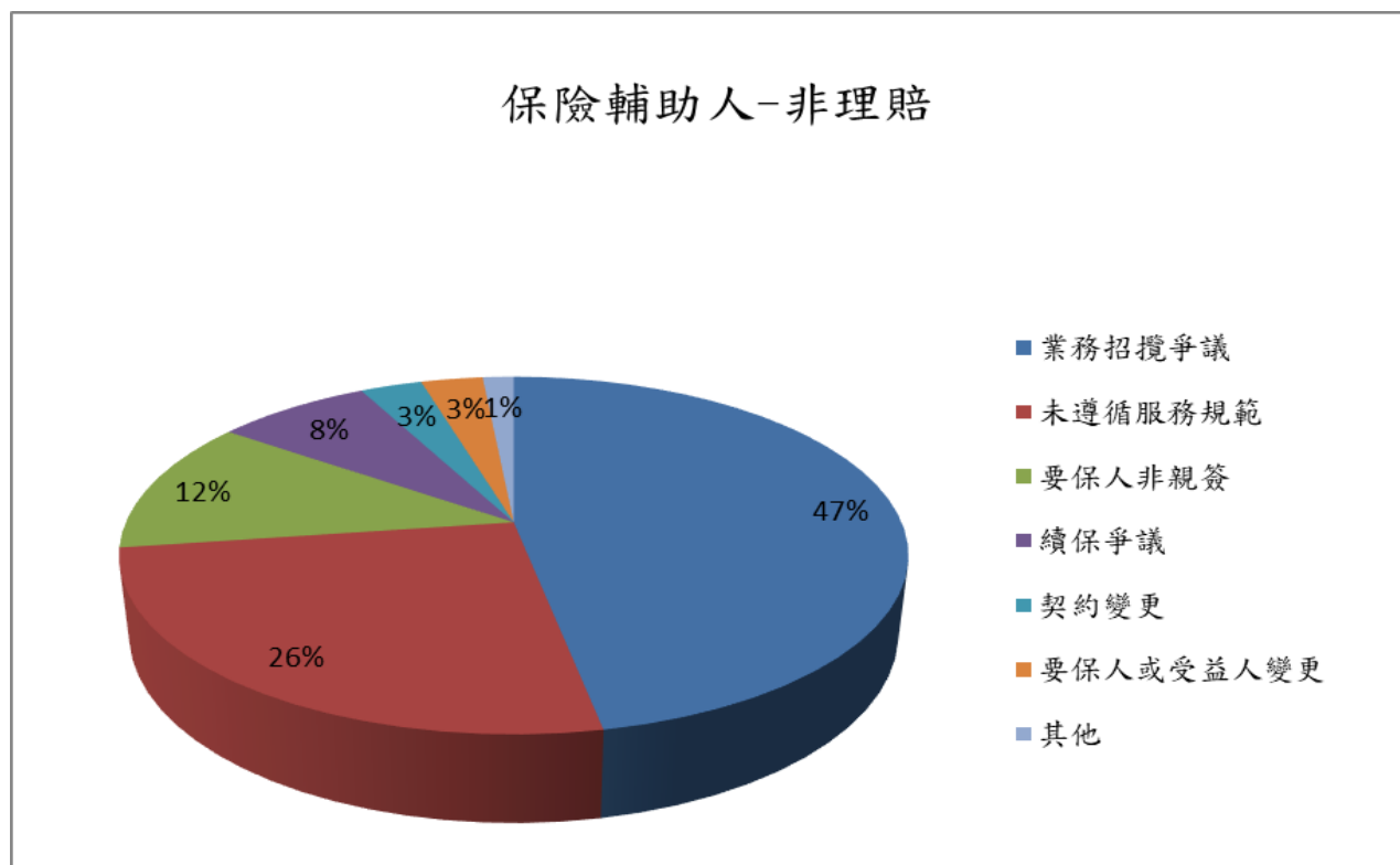
圖 15. 保險輔助人(非理賠類)常見爭議圓形圖
