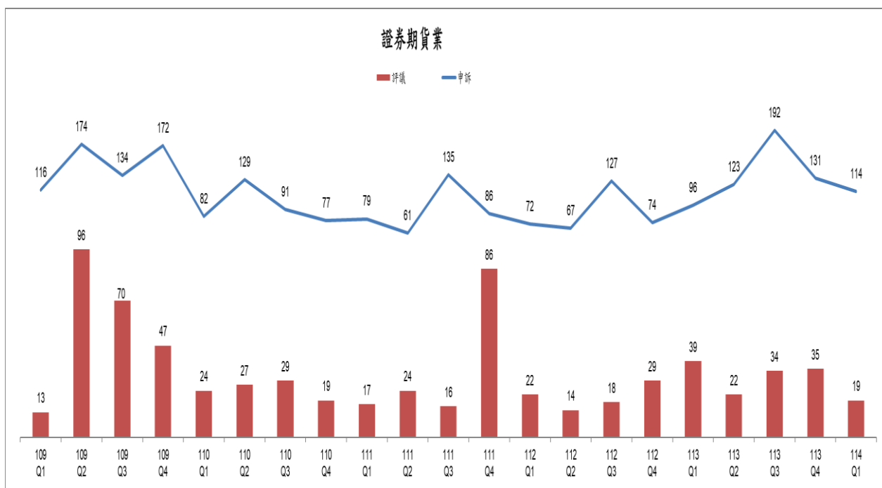
圖 8. 證券期貨業申訴暨評議案件數趨勢圖(季)
