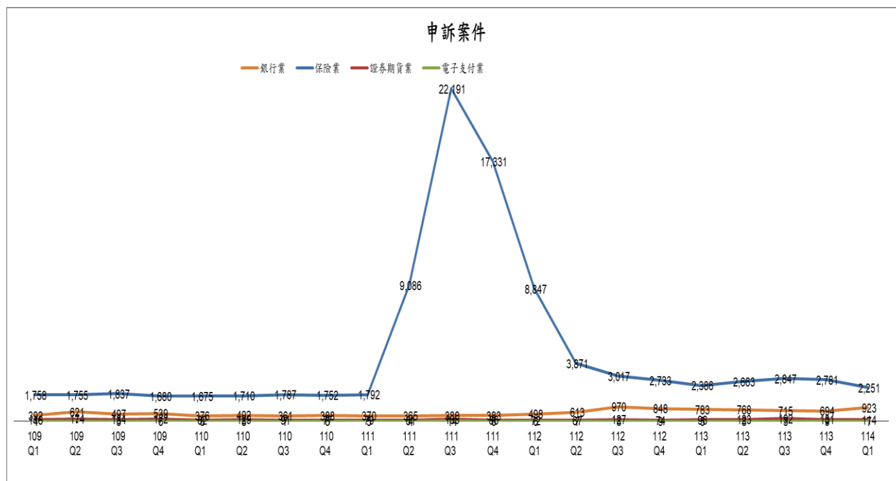
圖 2. 申訴案件數折線圖(全部業別)
