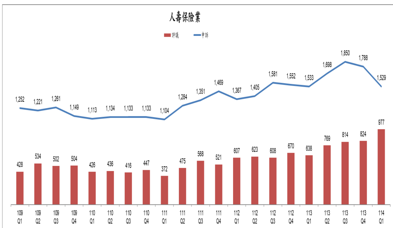
圖 5. 人壽保險業申訴暨評議案件數趨勢圖(季)
