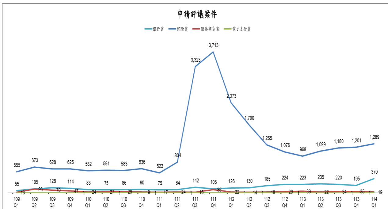
圖 3. 評議案件數折線圖(全部業別)
