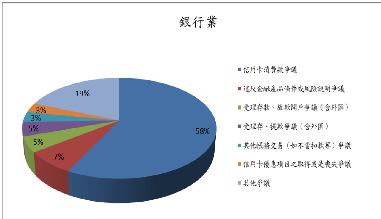
圖 10. 銀行業常見爭議圓形圖
