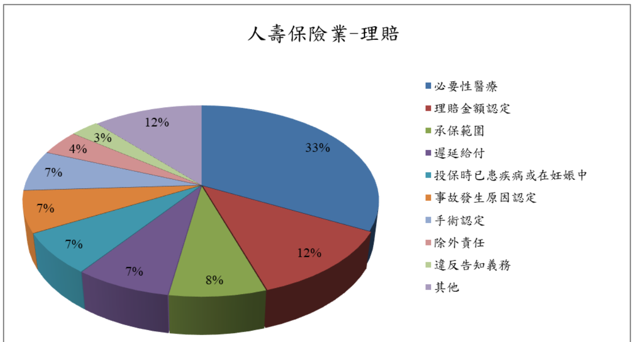
圖 11. 人壽保險業(理賠類)常見爭議圓形圖
