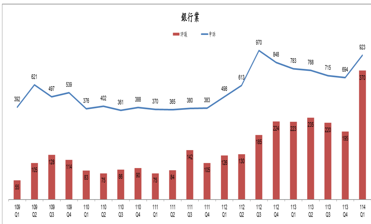
圖 4. 銀行業申訴暨評議案件數趨勢圖(季)
