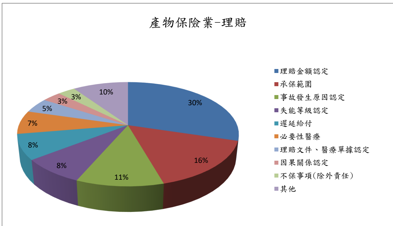
圖 13. 產物保險業(理賠類)常見爭議圓形圖
