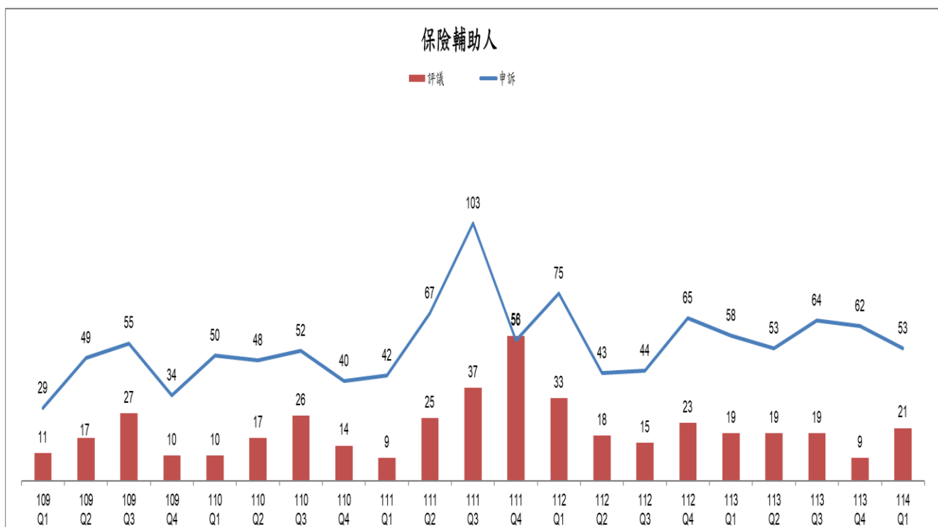
圖 7. 保險輔助人申訴暨評議案件數趨勢圖(季)
