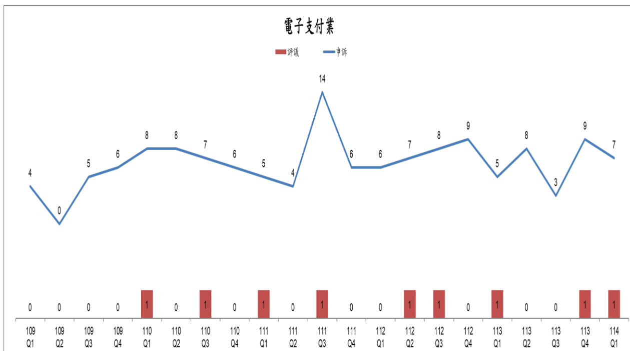
圖 9. 電子支付業申訴暨評議案件數趨勢圖(季)
