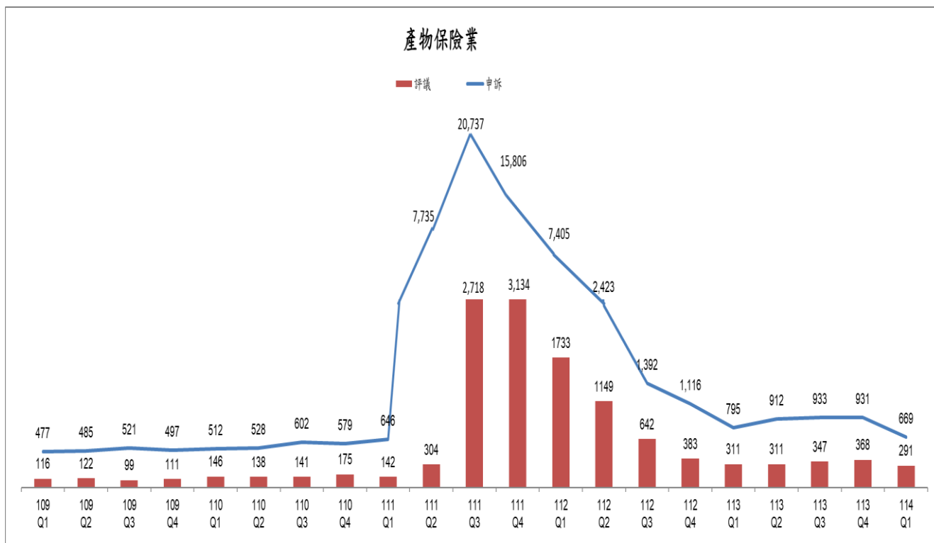
圖 6. 產物保險業申訴暨評議案件數趨勢圖(季)
